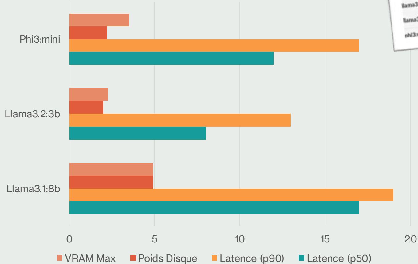
Benchmark LLMs
